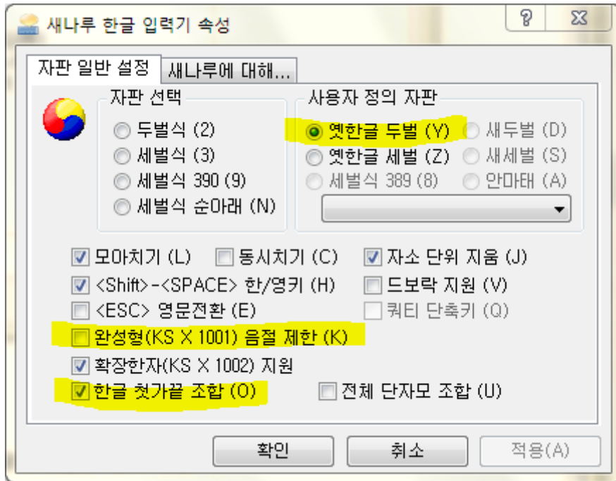
그림 1: 새나루 설정
